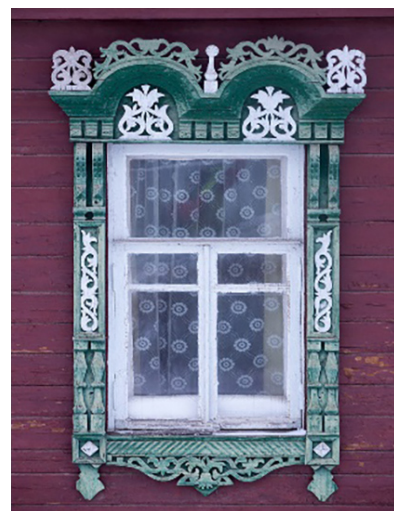
Рис. 3. Костромский наличник
